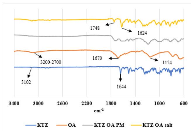
Fig. 8. FTIR spectra of bulk KTZ, OA, KTZ-OA physical mixture and KTZ-OA salt
